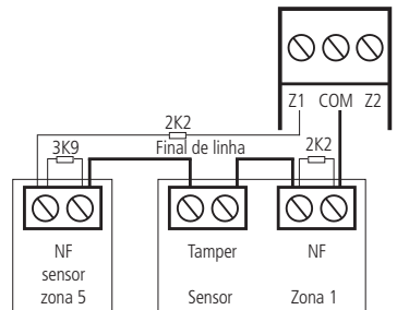
Ligação para um sensor com tamper (Zona 1) e um sensor sem tamper (Zona 5)
