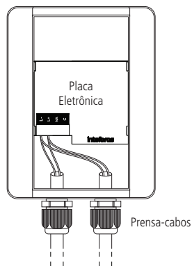
Instalação com prensa-cabos
