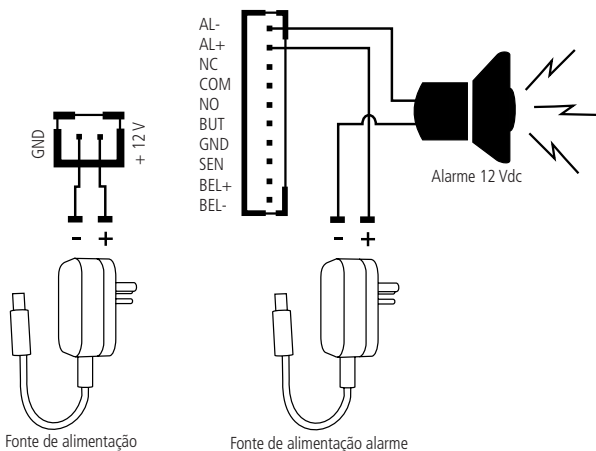
Ligação saída alarme
