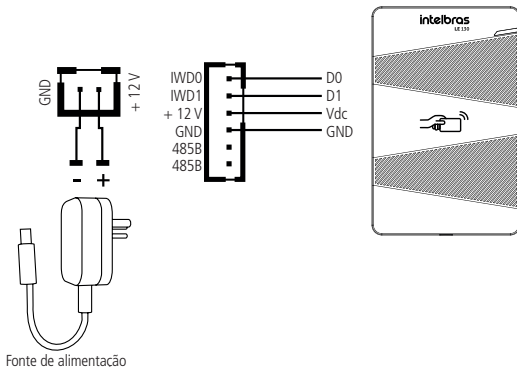
Ligação leitor auxiliar
