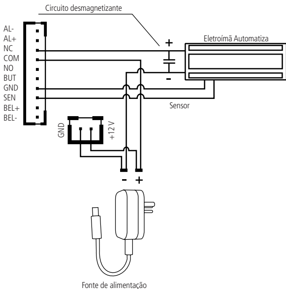
Ligação fechadura-eletrôimã Automatiza
