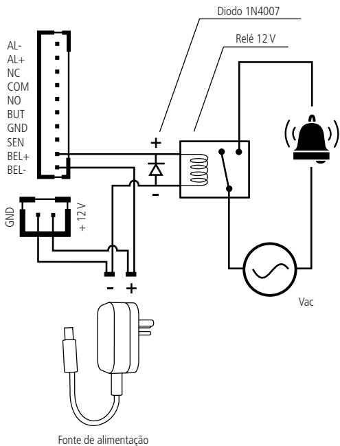
Ligação campainha 110/220 Vac
