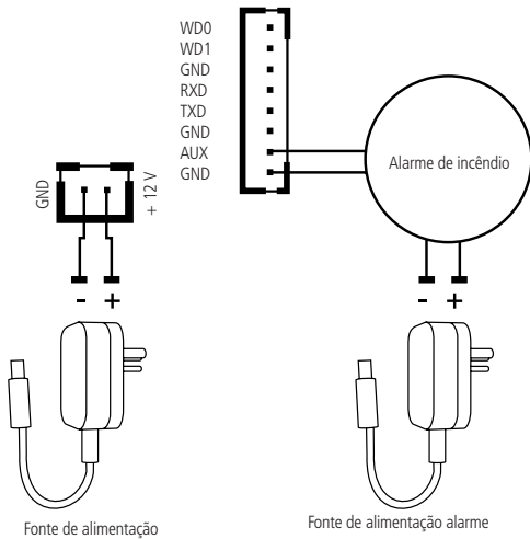
Ligação entrada auxiliar
