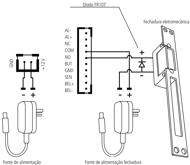
Ligação fechadura eletromecânica
