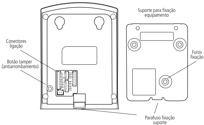
Fixação Duo SS 230 / Duo SS 230 MF
