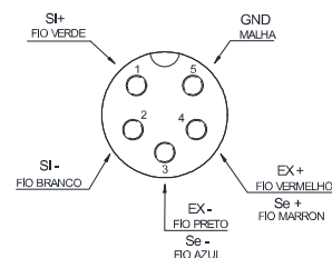
CONECTOR FÊMEA / CÉLULA
