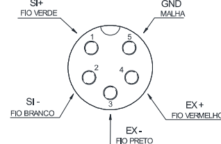
CONECTOR FÊMEA / CÉLULA
