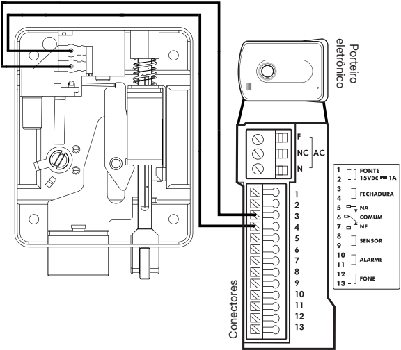
Fechadura ligada a um porteiro eletrônico
