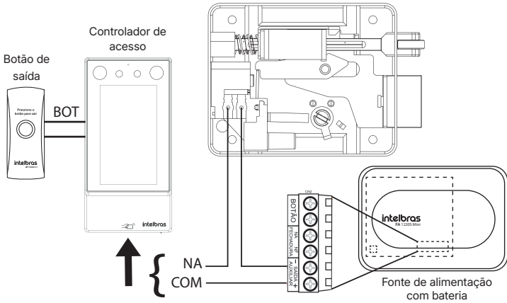
Fechadura ligada a um controle de acesso
