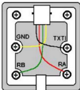
Tomada para instalação do TI 830i
