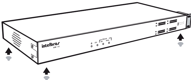
Fijación de los pies de goma en el producto
