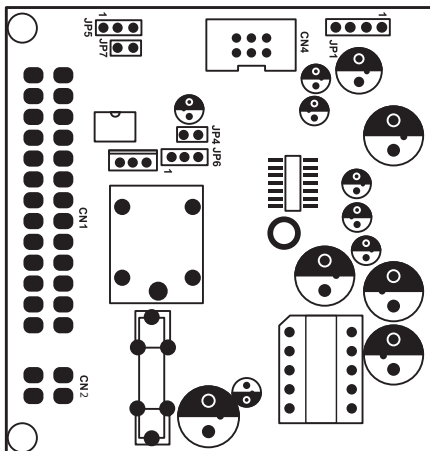
Placa base
