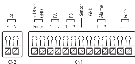
Bornes de ligação porteiro
