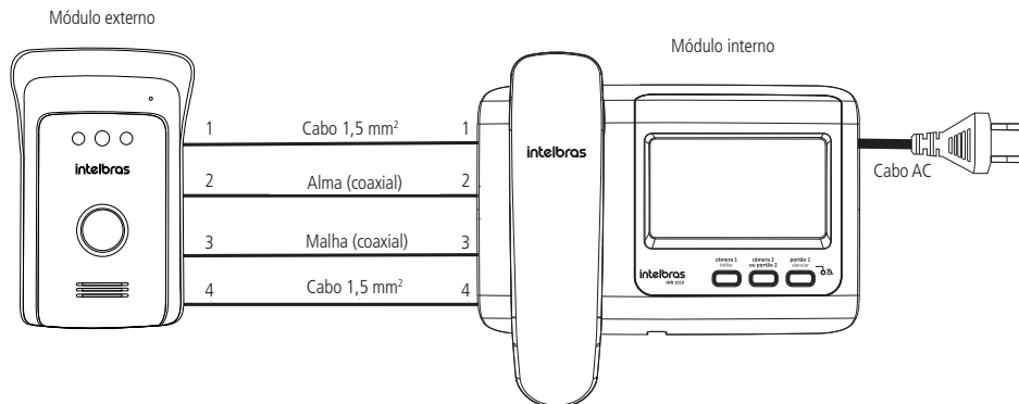
Instalação com cabo coaxial
