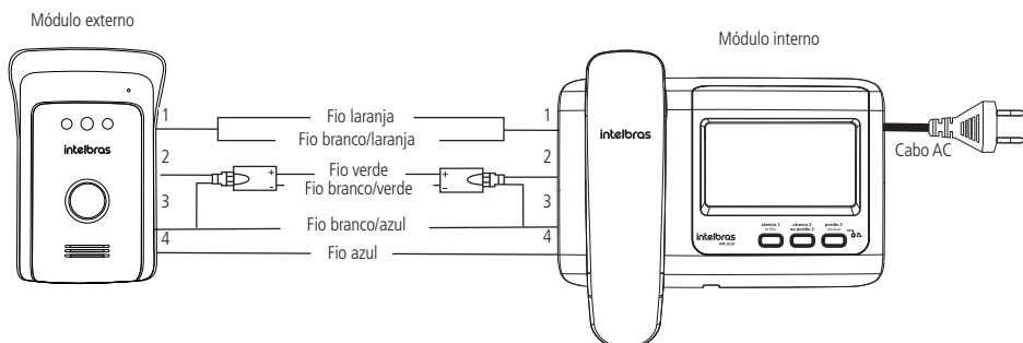
Instalação até 50 metros com balun
