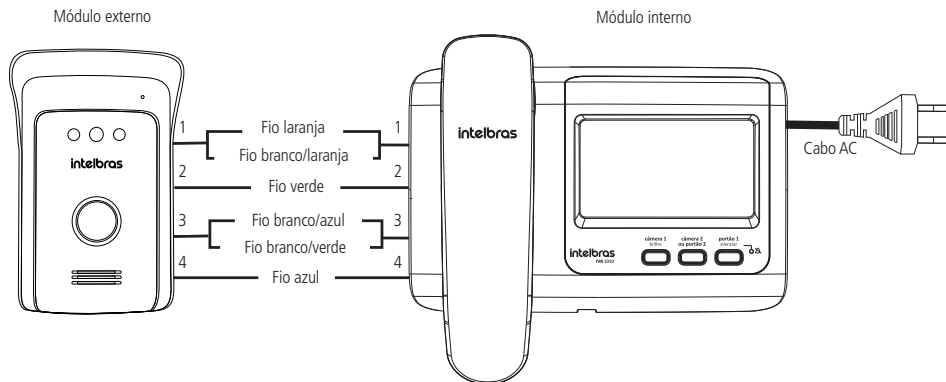
Instalação até 50 metros
