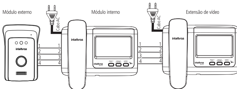
Instalação de extensão de vídeo
