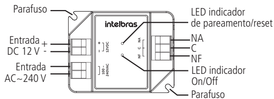
Visão frontal do Relé
