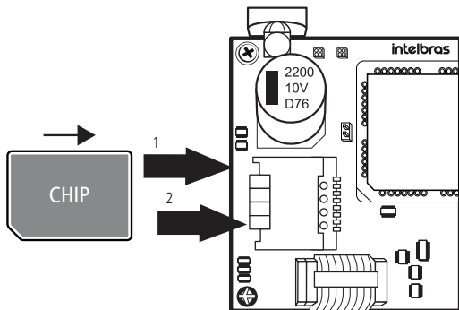
Alocação de chips no módulo GPRS XAG 8000
