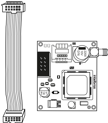
Módulo GPRS XAG 8000
