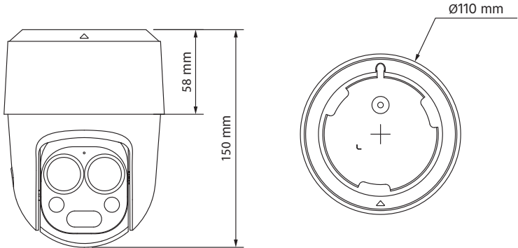
Vista detalhada
