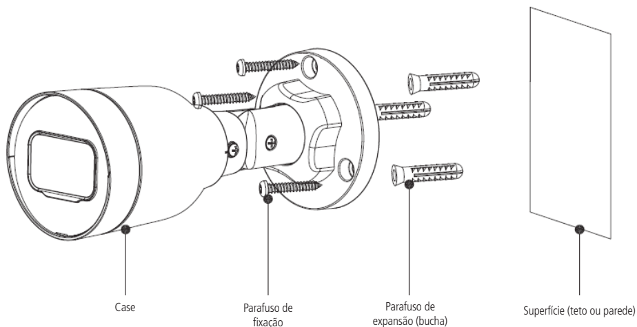
Vista detalhada VIP 3220 B
