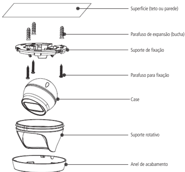
Vista detalhada VIP 3220 D
