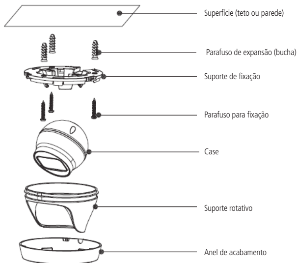
Vista detalhada VIP 1430 D
