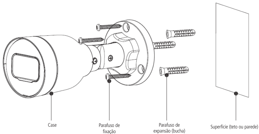
Vista detalhada VIP 1430 B
