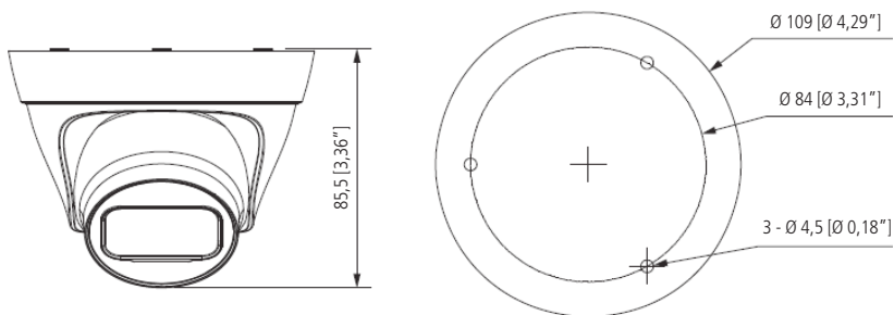
VIP 1430 D
