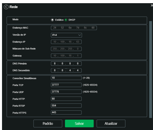
TCP/IP - versão 4
