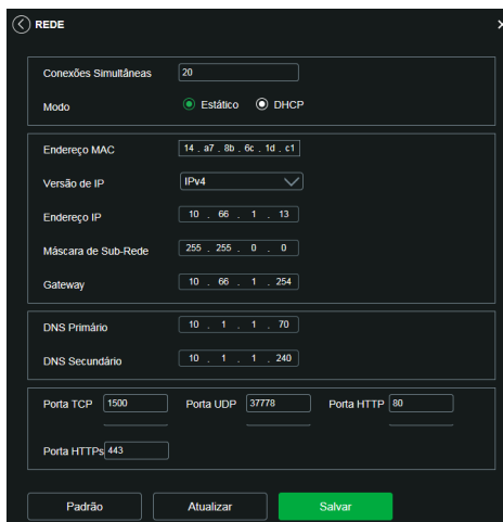
TCP/IP - versão 4
