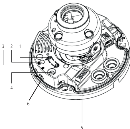
Descrição interna VIP 5450 D Z G2
