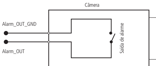
Esquema de saída de alarme VIP 5450 D Z G2
