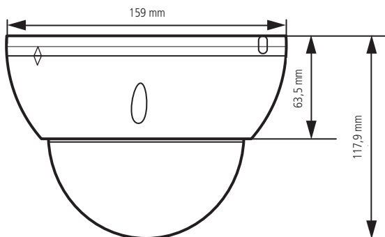
Vista lateral VIP 5450 D Z G2
