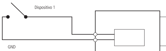
Esquema de entrada de alarme VIP 5450 D Z G2
