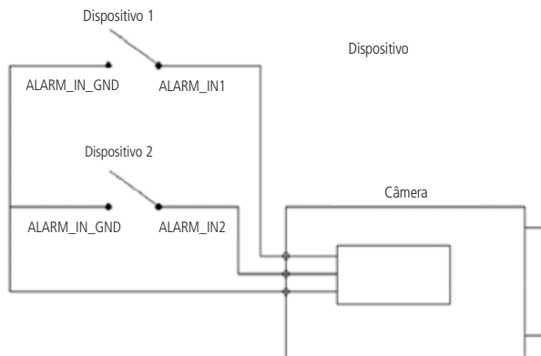
Esquema de entrada de alarme VIP 5450 Z G2
