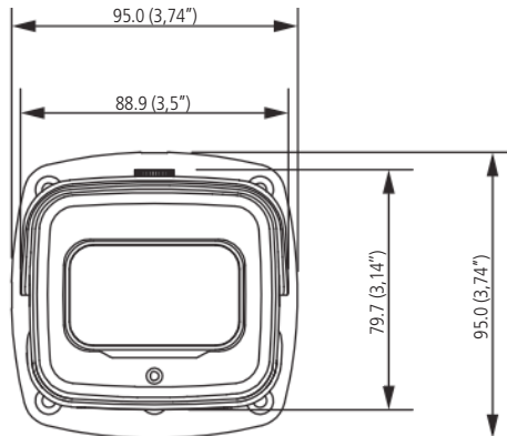
Visão frontal VIP 5450 Z G2
