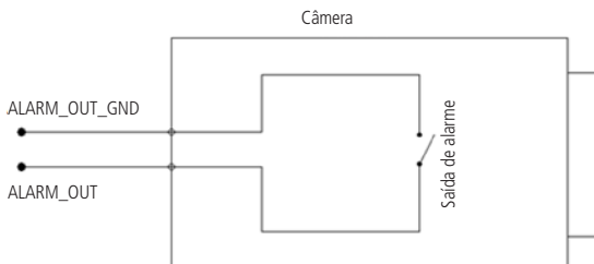
Esquema de saída de alarme VIP 5450 Z G2
