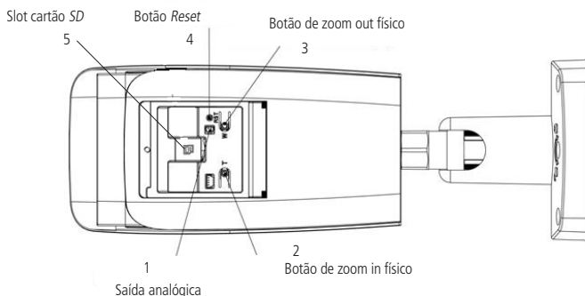
Visão inferior VIP 5450 Z G2
