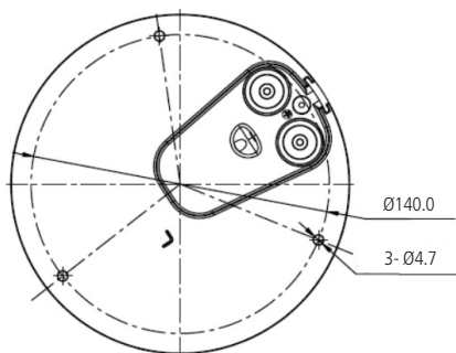
Vista frontal VIP 5450 D Z G2
