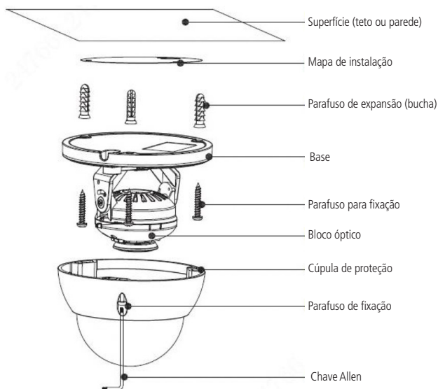
Vista detalhada VIP 3230 IK
