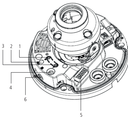
Descrição interna VIP 5550 DZ IA
