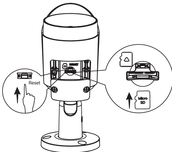
Acesso ao botão de Reset e microSD Card da VIP 3830 IA
