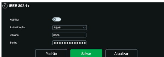
IEEE 802
