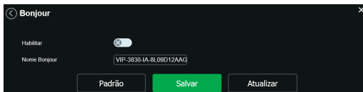
Bonjour
