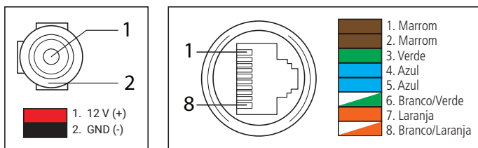
Cabo multifunções VIP 3830 IA
