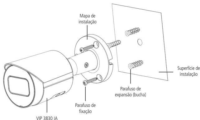
Vista detalhada VIP 3830 IA
