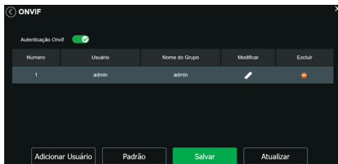
Onvif
