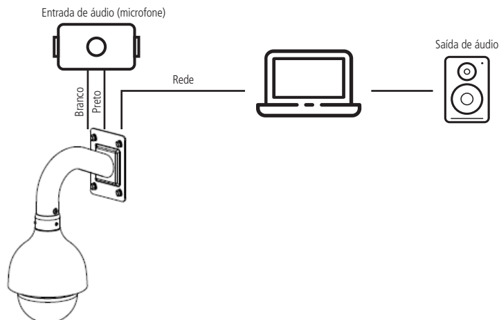
Conexão entrada de áudio da câmera
