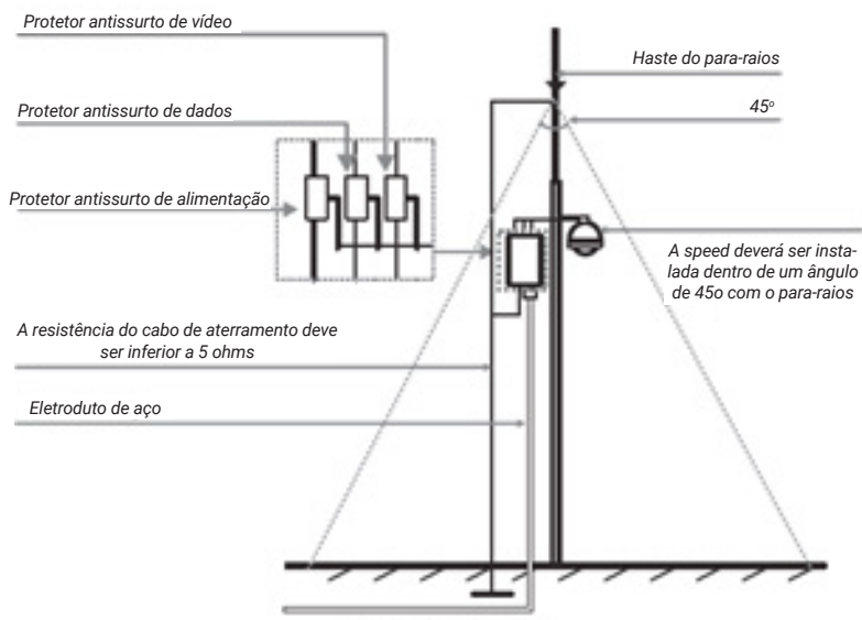
Instalação de segurança
