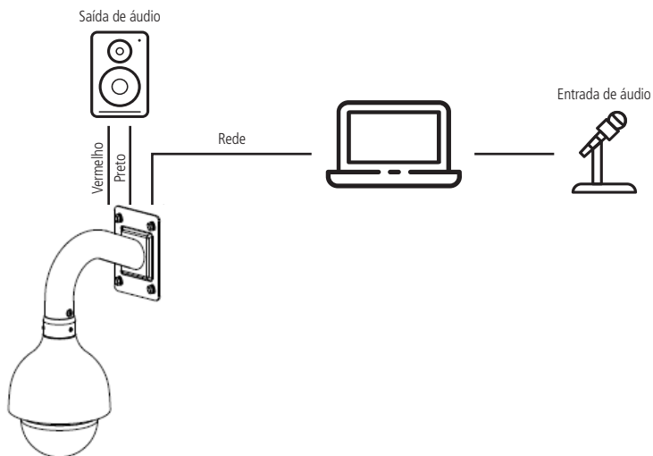
Conexão saída de áudio da câmera
