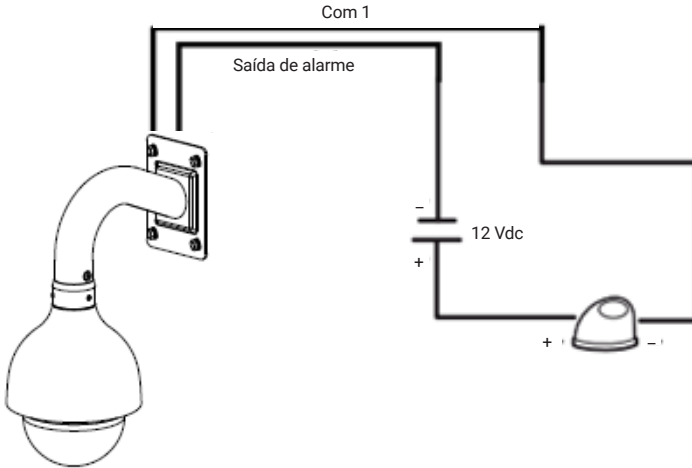
Conexão dos dispositivos de alarme
