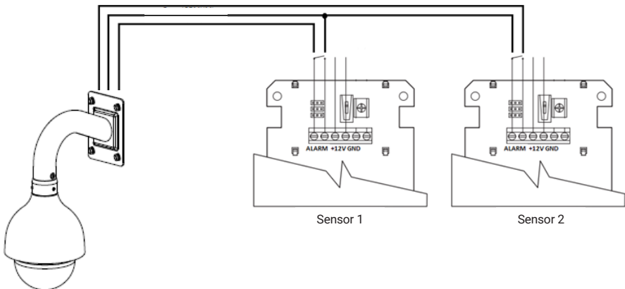
Conexão dos dispositivos de alarme
