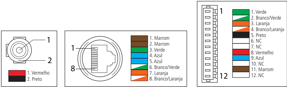
Cabo multifunções VIPW 1230 B e VIPW 1230 D
