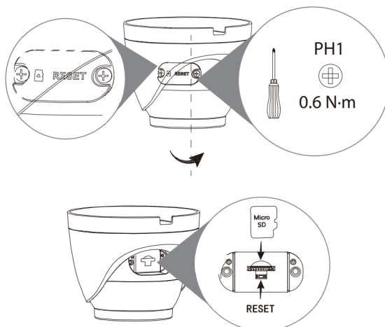
Acesso ao Botão de Reset e SD Card da VIPW 1230 D
