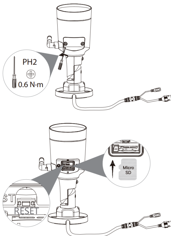
Acesso ao Botão de Reset e SD Card da VIPW 1230 B
