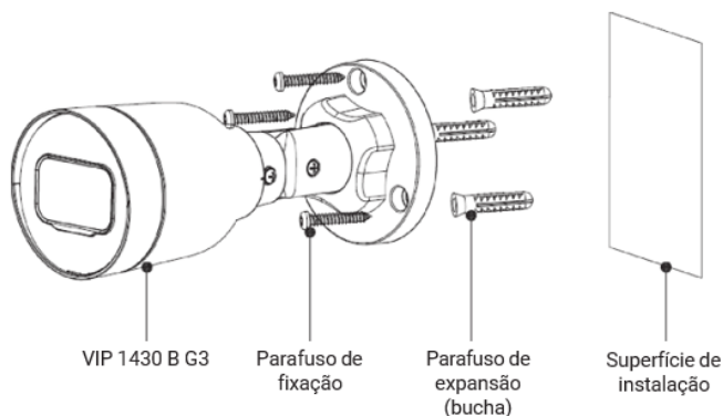
Vista detalhada VIP 1430 B G3
