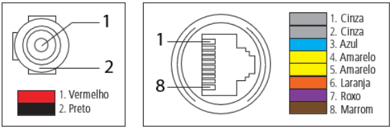
Cabo multifunções VIP 1430 B G3
