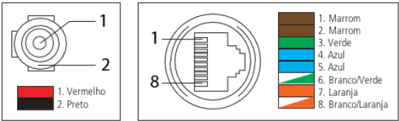
Cabo multifunções VIP 1430 D G3
