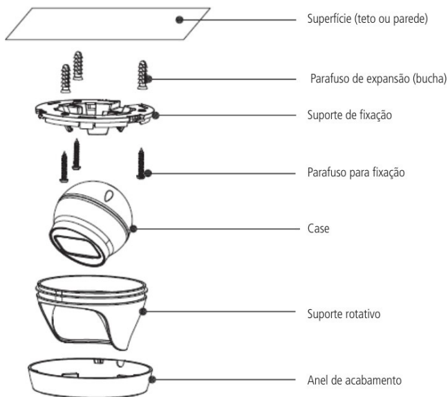
Vista detalhada VIP 1430 D G3
