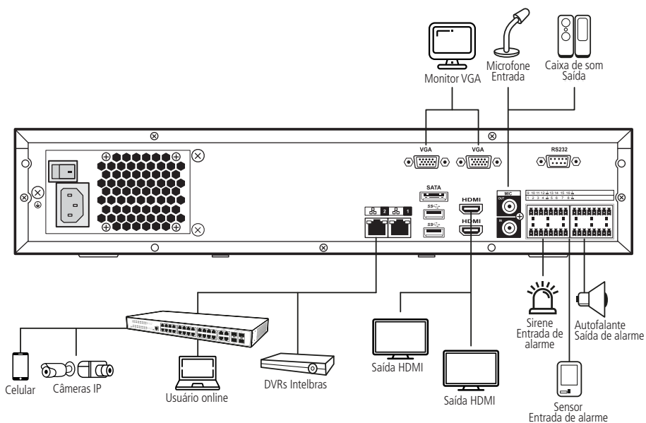
Exemplo de conexão - NVD 5124 P
