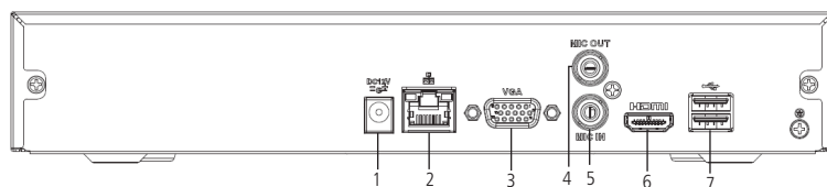
Painel posterior
