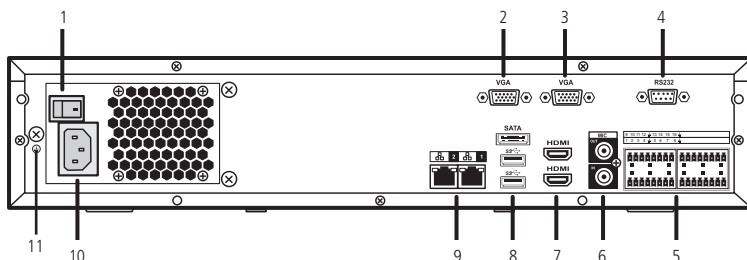
Panela posterior
