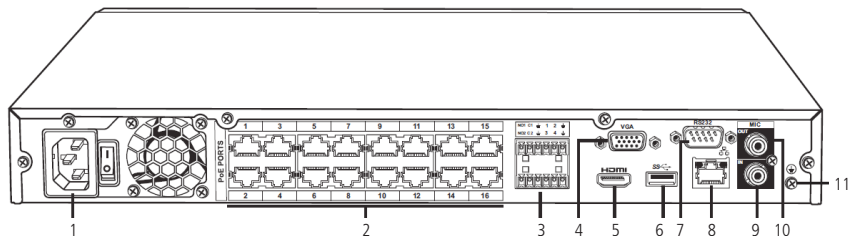
Painel posterior
