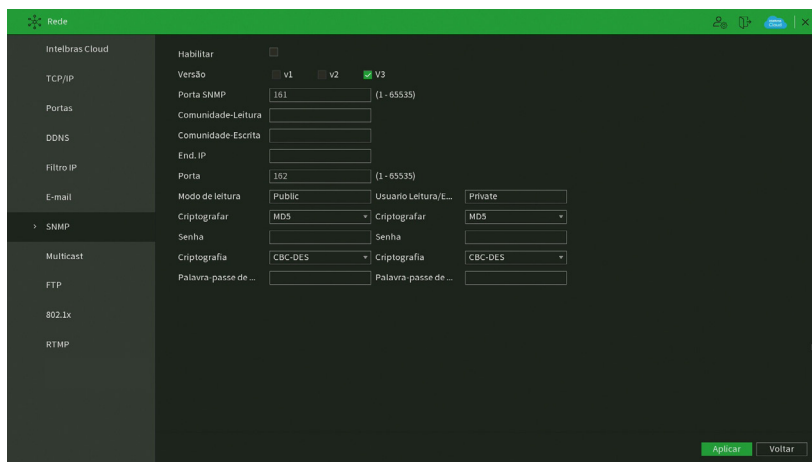
Menu SNMP
