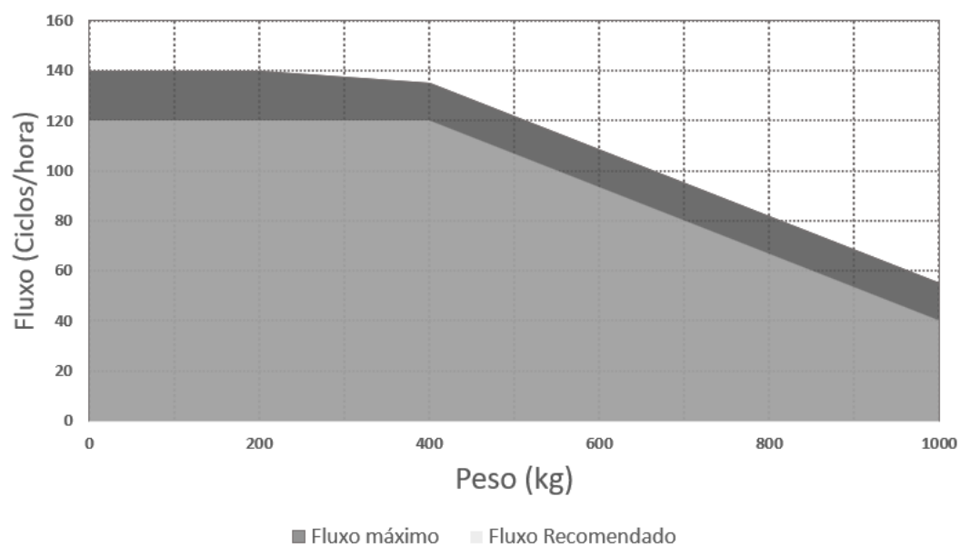
Curva de Peso vs. Ciclo Máximo
