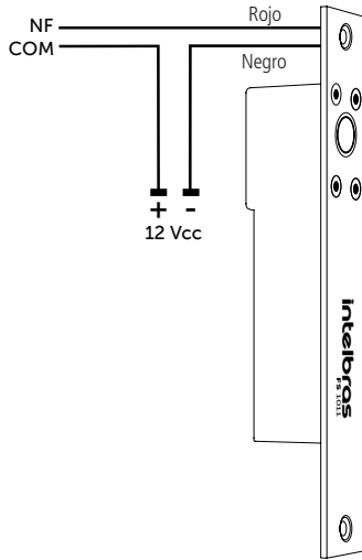
Solenoide FA 1011
