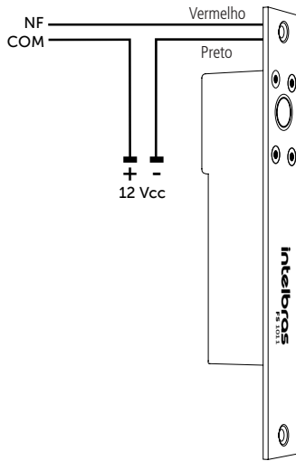
Solenoide FA 1011
