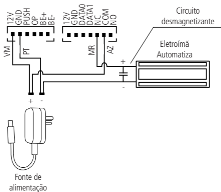
Ligação fechadura-eletrôímã Automatiza
