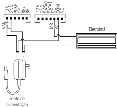
Ligação fechadura-eletrôimã
