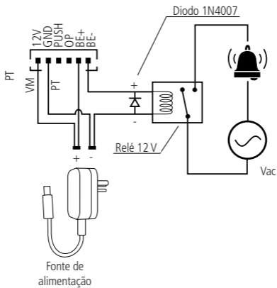
Ligação campainha
