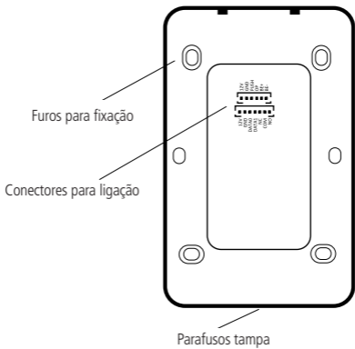
Imagem fixação Digiprox SA 203
