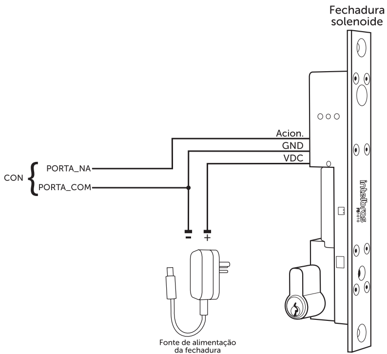
Exemplo de ligação de fechadura solenoide
