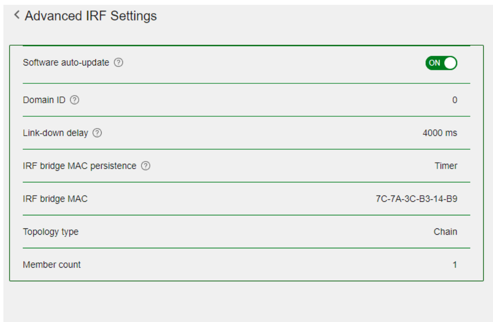
Figura 68 - Alterando o ID de Domínio IRF
