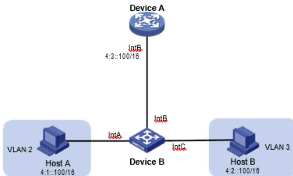
Figura 7 Ambiente de aplicação do ND Proxy local
