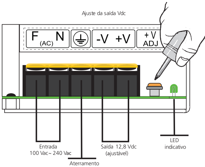
Visão frontal
