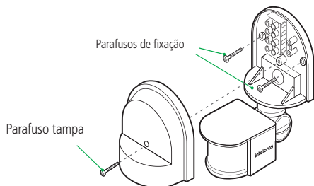
Fixação e instalação do sensor ESP 180 AE
