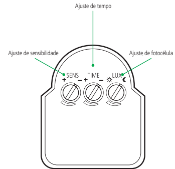
Trimpots de configurações
