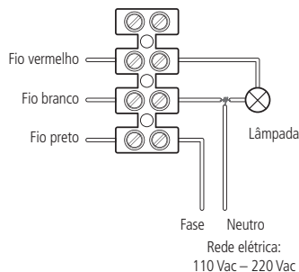
Conexões elétricas
