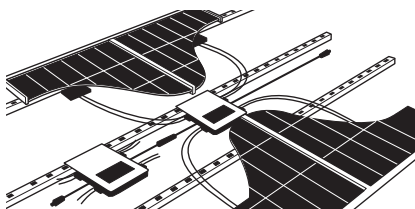
EGT 1200 MICRO conectado em paralelo
