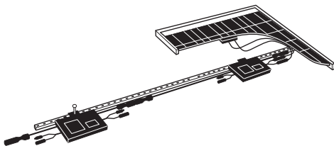
EGT 600 MICRO conectado em paralelo
