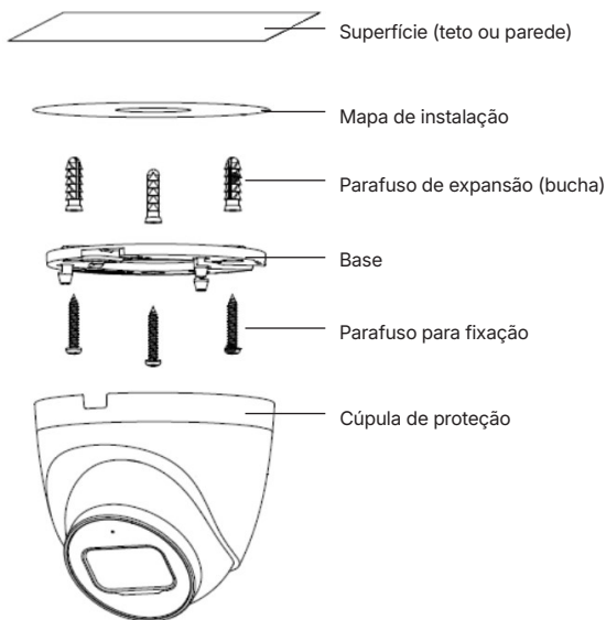
Vista detalhada VIP 3230 D FC+ IA
