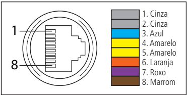
Cabo multifunções VIP 3230 FC+ IA
