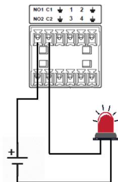
Conexão saída de alarme
