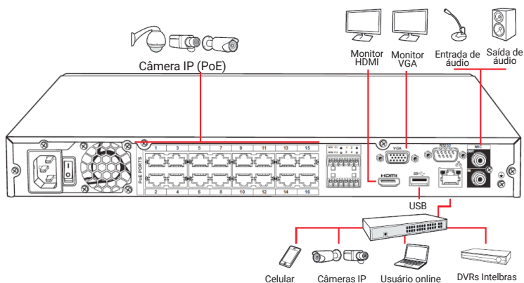
Exemplo de conexão
