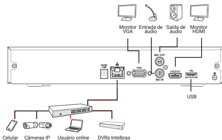
Exemplo de conexão
