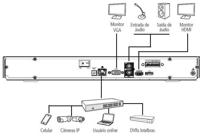
Exemplo de conexão
