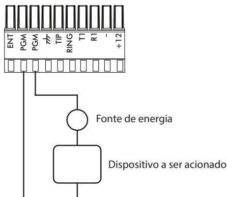
Imagem 10 – Ligando uma carga a saída PGM do GPRS 1000 UN
