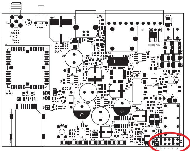
Imagem 13 – Placa GPRS 1000 UN
