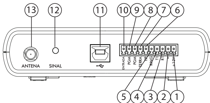
Imagem 04 – Parte traseira do GPRS 1000 UN
