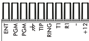
Imagem 05 – Conector tipo engate rápido
