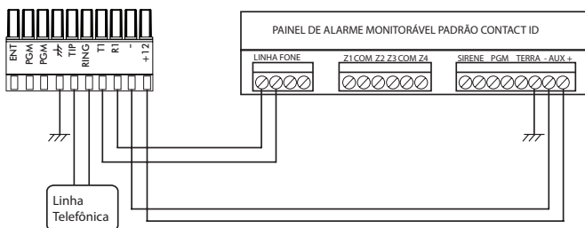
Imagem 07 – Conexão do GPRS 1000 UN com painel de alarme
