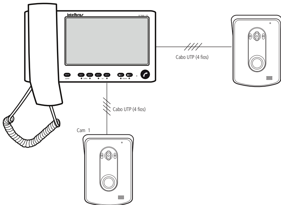
Instalação com 1 módulo interno e 2 módulos externos
