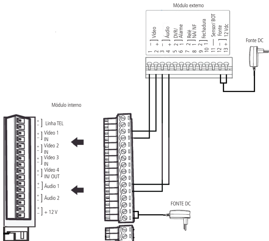
Instalação básica com fonte DC
