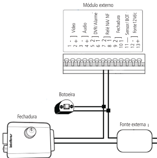
Instalação de botoeira na fechadura 2
