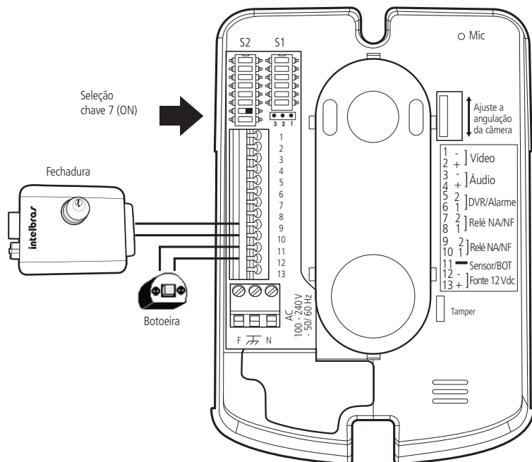
Instalação de fechadura com botoeira
