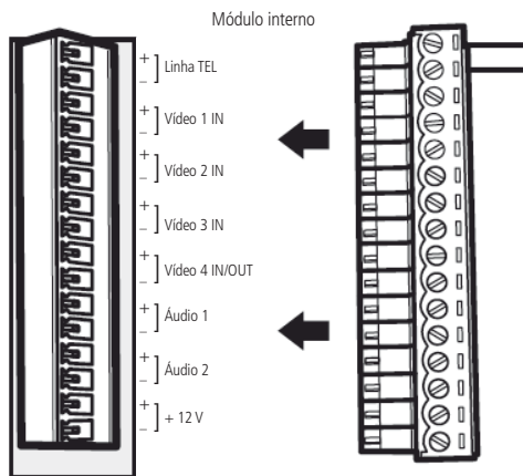
Instalação da linha telefônica
