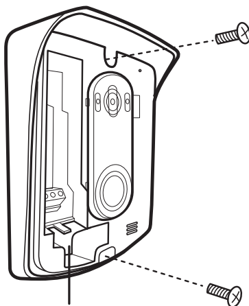
Passagem de cabos
