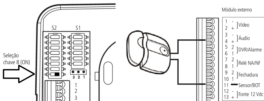
Instalação de sensor
