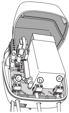
a. Cabo da saída de alta tensão; b. Cabo de aterramento; c. Cabo de retorno de alta tensão.
